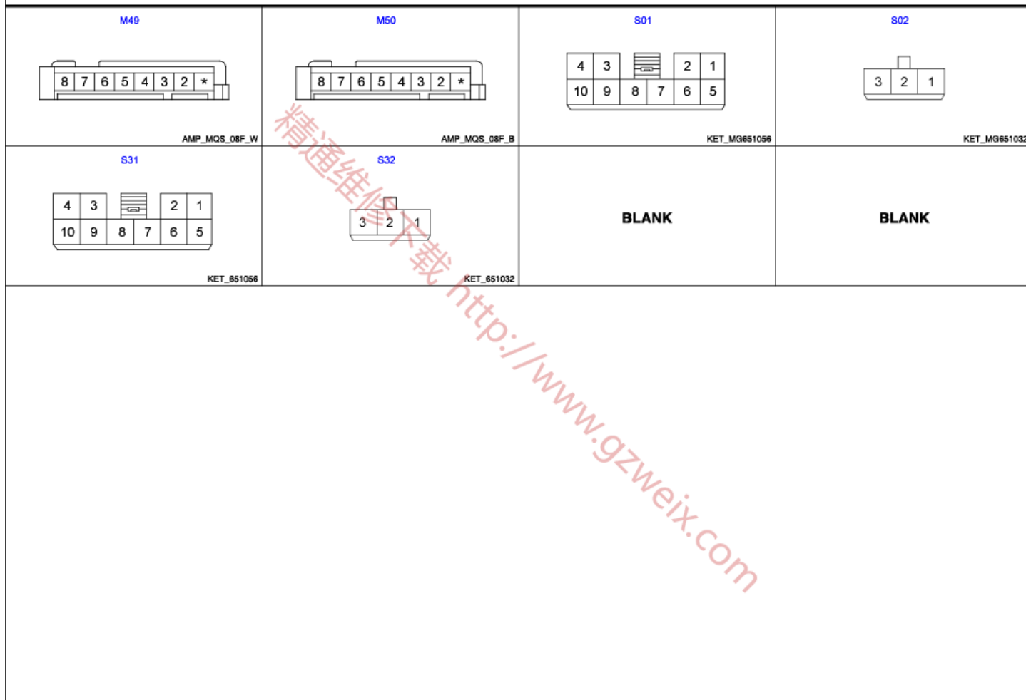
电动座椅加热器系统 (3)
